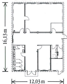
Basis-Modul 1 für den 1gruppigen Kindergarten.
