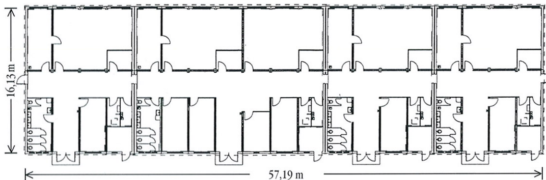
3 Basis-Module 1 und 1 Basis-Modul 2 für den 4gruppigen Kindergarten.
