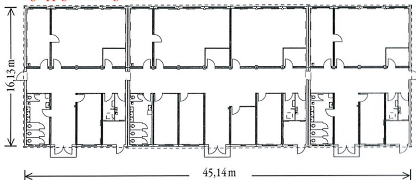
2 Basis-Module 1 und 1 Basis-Modul 2 für den 3gruppigen Kindergarten.
