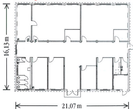
Basis-Modul 2 für den 1gruppigen Kindergarten mit Mehrzweckraum.
