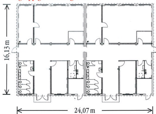
2 Basis-Module 1 für den 2gruppigen Kindergarten.
